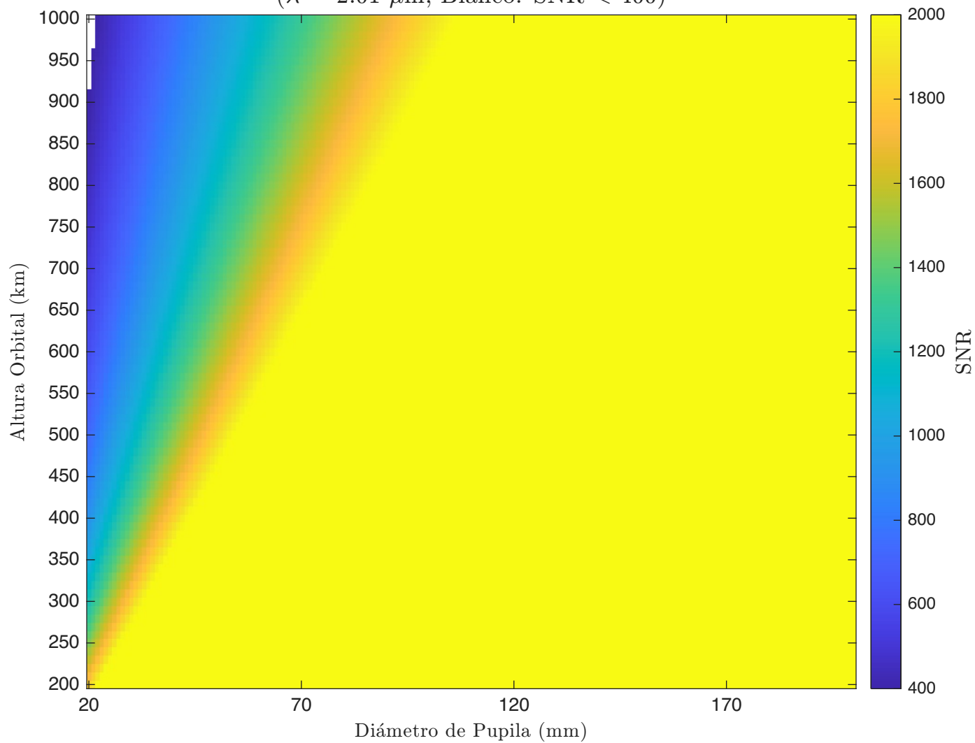
SNR - Cassegrain - Detector 3 ( \lambda = 2.01 \mu\text{m} , Blanco: SNR < 400)
